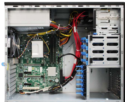
TWR-1213-7S-USB30 Vista dall'alto senza parete laterale
