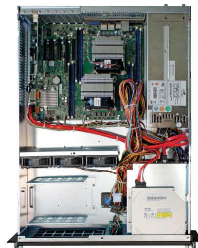
GO-215V Vista frontale senza copertura superiore
