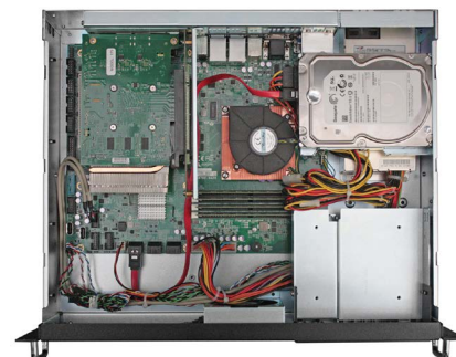
GOI-252H: Vista dall'alto - Riser 7° slot
