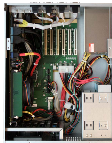
GOMI-610 Vista dall'alto senza copertura superiore
