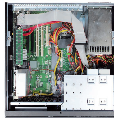
GO-120SR Vista dall'alto senza copertura superiore
