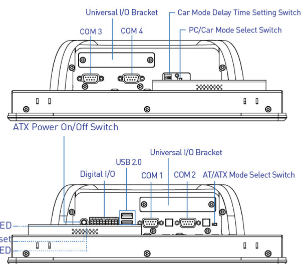
Left I/O
