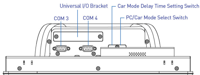
Right I/O
