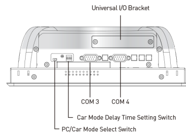
Right I/O
